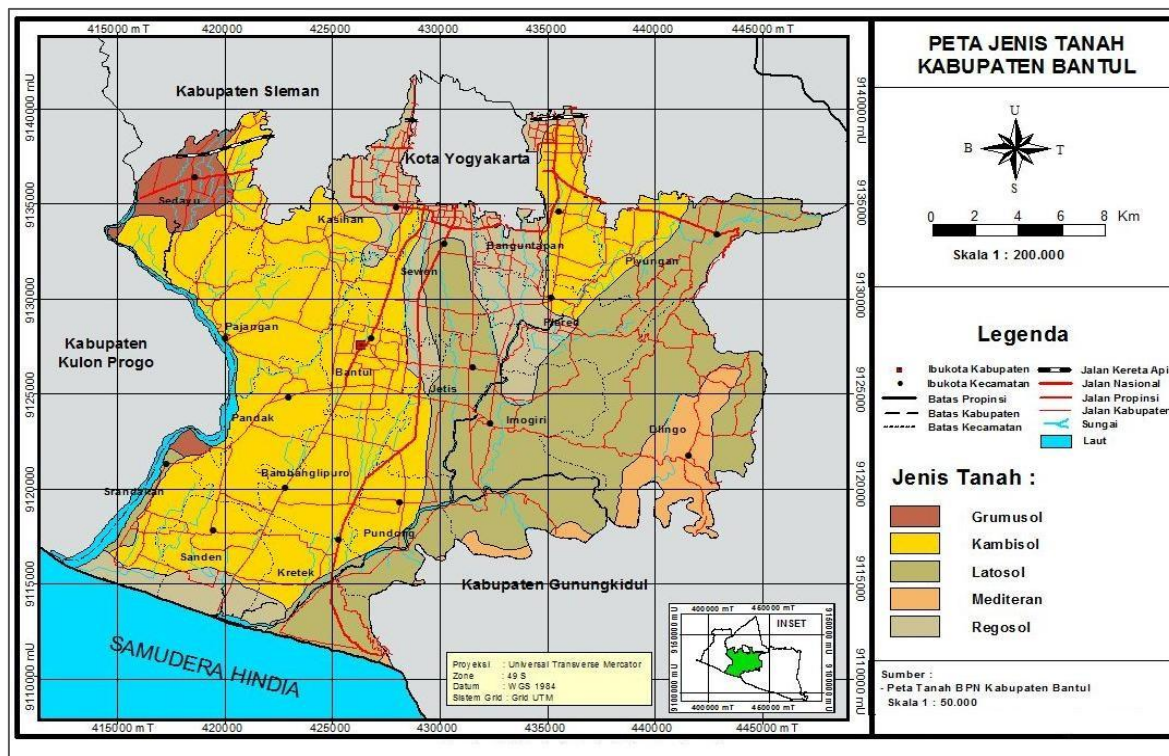
Gambar 2.6 Peta Jenis Tanah Kabupaten Bantul
