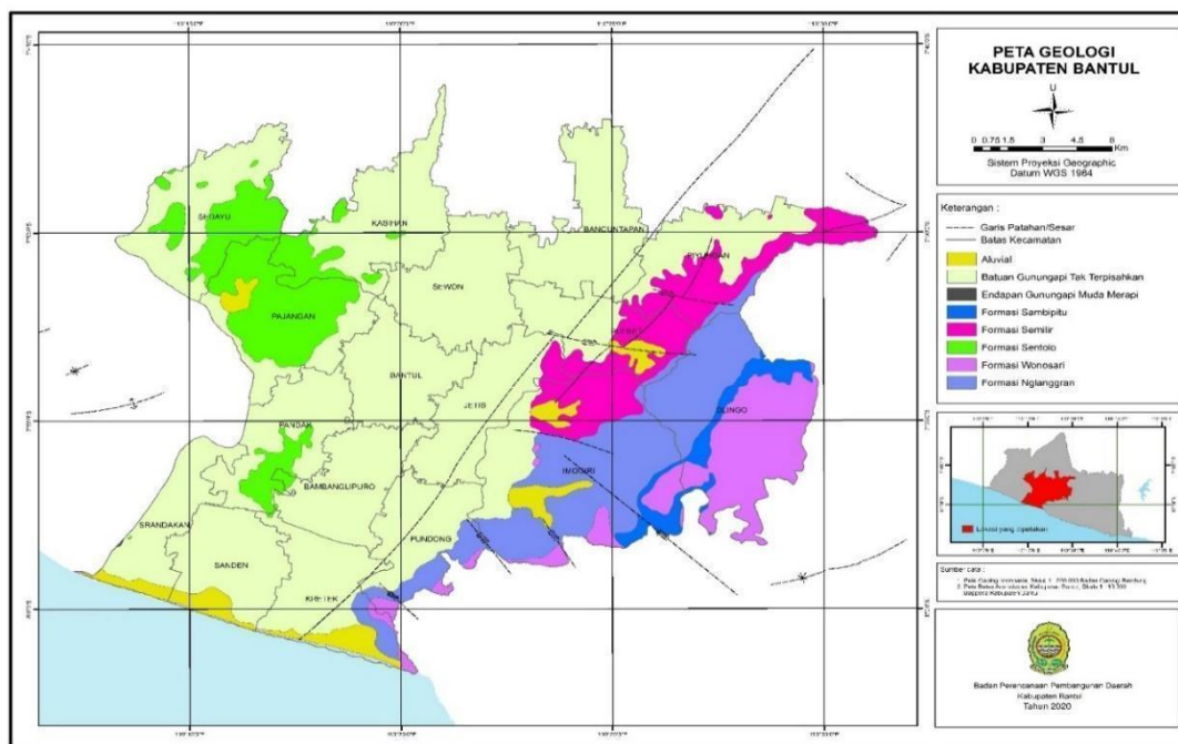
Gambar 2.5 Peta Geologi Kabupaten Bantul
