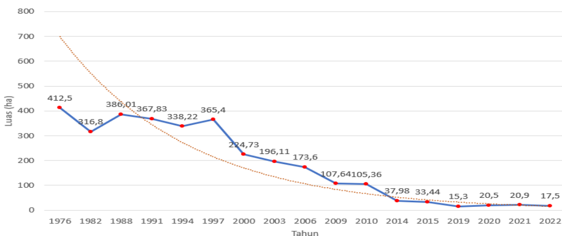
Gambar 2.11 Pengurangan Luas Area Pasir Terbuka di Zona Inti dan Penyangga Gumuk Pasir Parangtritis
